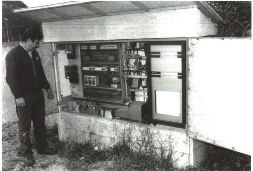
Hier sehen wir Benno Jäger beim Pumpwerk II (Nähe Sportplatz). Hier befinden sich zwei Abwassertauchpumpen mit einer Leistung von je 60 Liter/sec. und einer Förderhöhe von 4.20 Meter. Im Normalfall wird das Dränwasser aufgestaut und überläuft in den Vorfluter, die Esche. Zur Steuerung der Schieber und der Pumpen werden die Wasserstände der Esche laufend gemessen und registriert.
