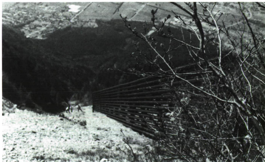
Um den Wald vor Steinschlägen zu schützen, ist unter grossem Einsatz, eine 52 Meter lange und 4 Meter hohe Ablenk- wand aus Eisen aufgestellt worden. Mit diesem Bauwerk werden die zu Tal stürzenden Steine direkt in den Rüfekanal geleitet
